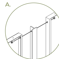
PŘIPOJENÍ STŘEDOVÉHO SLOUPKU
