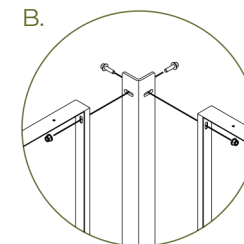
PŘIPEVNĚNÍ ROHOVÉHO SLOUPKU
