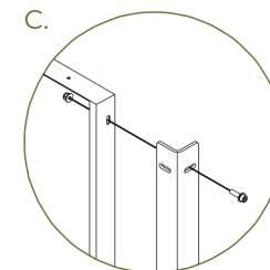
PŘIPOJENÍ ROHŮ NA OKRAJI
